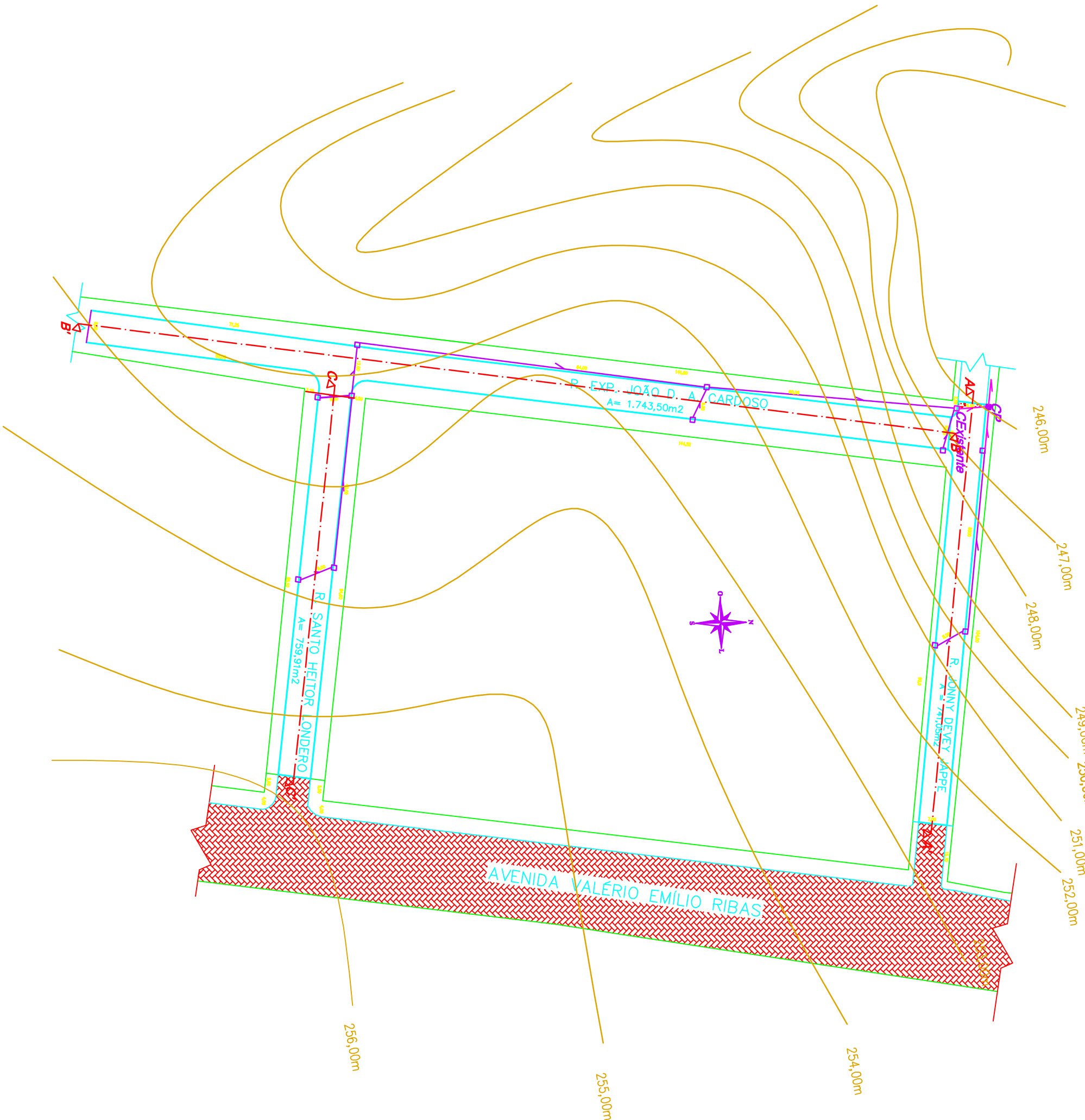
PLANTA PLANIALTIMÉTRICA Esc. 1/500
