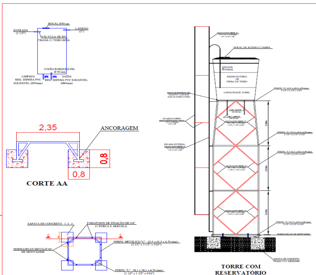
PLANTA BAIXA PLATAFORMA DE APOIO (BASE DO RESERVATÓRIO)
