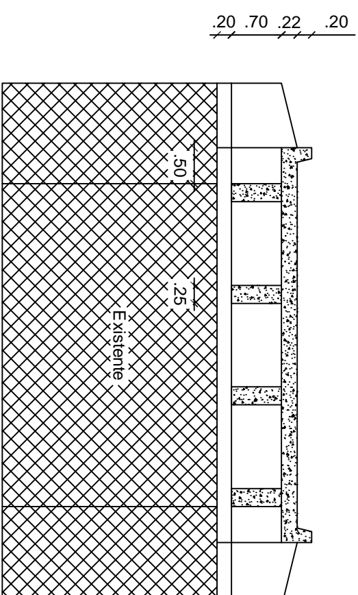
Corte BB
