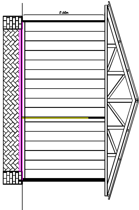
CORTE AA' ESC. 1/50
