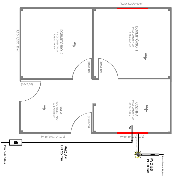
PLANTA DAS INST. HIDROSSANITÁRIAS ESC. 1/50
