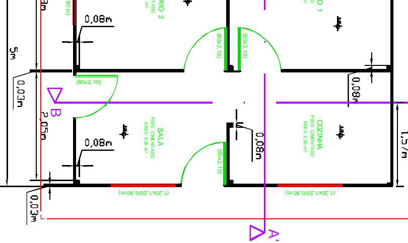
PLANTA BAIXA ESC. 1/50
